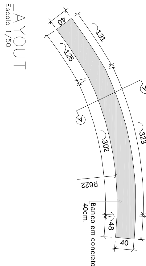
DETALHAMENTO BANCO 02
